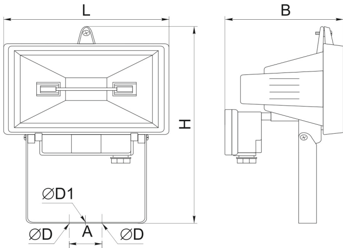
Рисунок 1. Габаритные и установочные размеры прожекторов ИО 150, ИО 500, ИО 1000, ИО 1500
